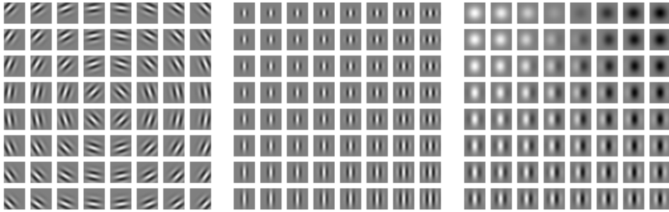
图 9.18: 具有各种参数设置的 Gabor 函数。白色表示绝对值大的正权重，黑色表示绝对值大的负权重，背景灰色对应于零权重。(左) 控制坐标系的参数具有不同值的 Gabor 函数，这些参数包括： x_0 、 y_0 和 \gamma 。在该网格中的每个 Gabor 函数被赋予和它在网格中的位置成比例的 x_0 和 y_0 的值，并且 \tau 被选择为使得每个 Gabor 过滤器对从网格中心辐射出的方向非常敏感。对于其他两幅图， x_0 、 y_0 和 \gamma 固定为零。(中) 具有不同高斯比例参数 \beta_x 和 \beta_y 的 Gabor 函数。当我们从左到右通过网格时，Gabor 函数被设置为增加宽度（减少 \beta_x ）；当我们从上到下通过网格时，Gabor 函数被设置为增加高度（减少 \beta_y ）。对于其他两幅图， \beta 值固定为图像宽度的 1.5 倍。(右) 具有不同的正弦参数 f 和 \phi 的 Gabor 函数。当我们从上到下移动时， f 增加；当我们从左到右移动时， \phi 增加。对于其他两幅图， \phi 固定为 0， f 固定为图像宽度的 5 倍。
