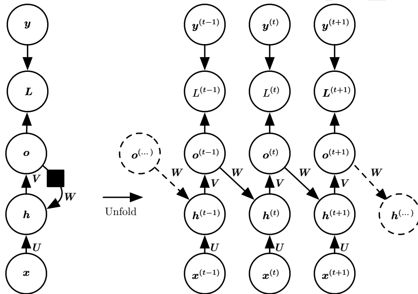
图 10.4: 此类 RNN 的唯一循环是从输出到隐藏层的反馈连接。在每个时间步 t ，输入为 x_t ，隐藏层激活为 h^{(t)} ，输出为 o^{(t)} ，目标为 y^{(t)} ，损失为 L^{(t)} 。(左)回路原理图。(右)展开的计算图。这样的 RNN 没有图 10.3 表示的 RNN 那样强大（只能表示更小的函数集合）。图 10.3 中的 RNN 可以选择将其想要的关于过去的任何信息放入隐藏表示 h 中并且将 h 传播到未来。该图中的 RNN 被训练为将特定输出值放入 o 中，并且 o 是允许传播到未来的唯一信息。此处没有从 h 前向传播的直接连接。之前的 h 仅通过产生的预测间接地连接到当前。 o 通常缺乏过去的重要信息，除非它非常高维且内容丰富。这使得该图中的 RNN 不那么强大，但是它更容易训练，因为每个时间步可以与其他时间步分离训练，允许训练期间更多的并行化，如第 10.2.1 节所述。
