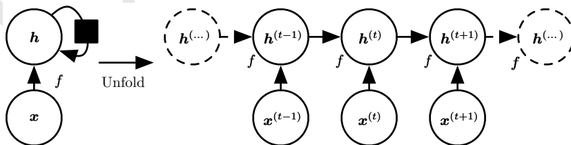
图 10.2: 没有输出的循环神经网络。此循环神经网络只处理来自输入 \mathbf{x} 的信息，将其合并到经过时间向前传播的状态 \mathbf{h} 。(左) 回路原理图。黑色方块表示单个时间步的延迟。(右) 同一网络被视为展开的计算图，其中每个节点现在与一个特定的时间实例相关联。
