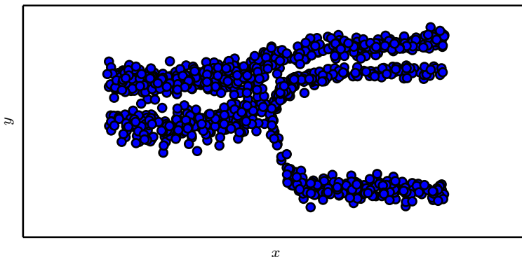
图 6.4: 从具有混合密度输出层的神经网络中抽取的样本。输入 x 从均匀分布中采样，输出 y 从 p_{\text{model}}(y | x) 中采样。神经网络能够学习从输入到输出分布的参数的非线性映射。这些参数包括控制三个组件中的哪一个将产生输出的概率，以及每个组件各自的参数。每个混合组件都是高斯分布，具有预测的均值和方差。输出分布的 these 方面都能够相对输入 x 变化，并且以非线性的方式改变。
