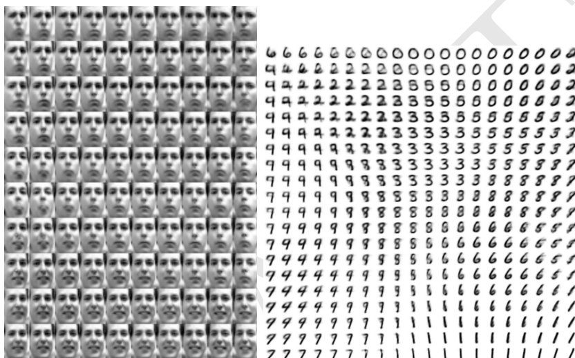
图 20.6: 由变分自编码器学习的高维流形在 2 维坐标系中的示例 (Kingma and Welling, 2014a)。我们可以在纸上直接绘制两个可视化的维度，因此可以使用 2 维潜在编码训练模型来了解模型的工作原理（即使我们认为数据流形的固有维度要高得多）。图中所示的图像不是来自训练集的样本，而是仅仅通过改变 2 维“编码” z ，由模型 p(x|z) 实际生成的图像 x （每个图像对应于“编码” z 位于 2 维均匀网格的不同选择）。(左) Frey 人脸流形的 2 维映射。其中一个维度（水平）已发现大致对应于面部的旋转，而另一个（垂直）对应于情绪表达。(右) MNIST 流形的 2 维映射。
