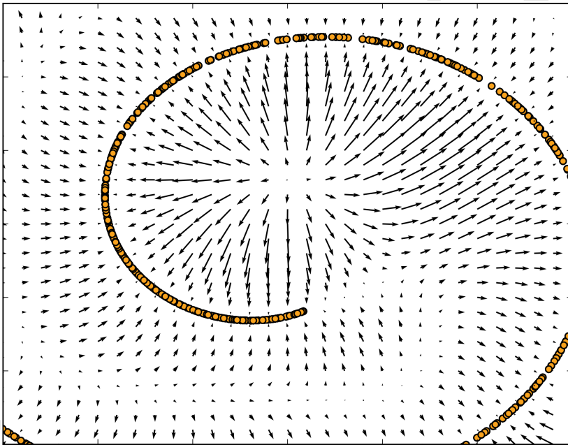
图 14.5: 由去噪自编码器围绕 1 维弯曲流形学习的向量场，其中数据集中在 2 维空间中。每个箭头与重构向量减去自编码器的输入向量后的向量成比例，并且根据隐式估计的概率分布指向较高的概率。向量场在估计的密度函数的最大值处（在数据流形上）和密度函数的最小值处都为零。例如，螺旋臂形成局部最大值彼此连接的 1 维流形。局部最小值出现在两个臂间隙的中间附近。当重构误差的范数（由箭头的长度示出）很大时，在箭头的方向上移动可以显著增加概率，并且在低概率的地方大多也是如此。自编码器将这些低概率点映射到较高的概率重构。在概率最大的情况下，重构变得更准确，因此箭头会收缩。经 Alain and Bengio (2013) 许可转载此图。
